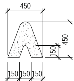
SECTION 'A'
