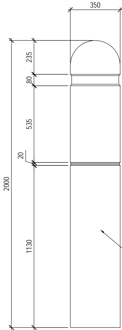
ELEVATION
