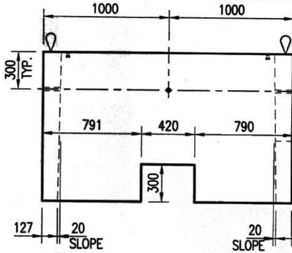
A ELEVATION
