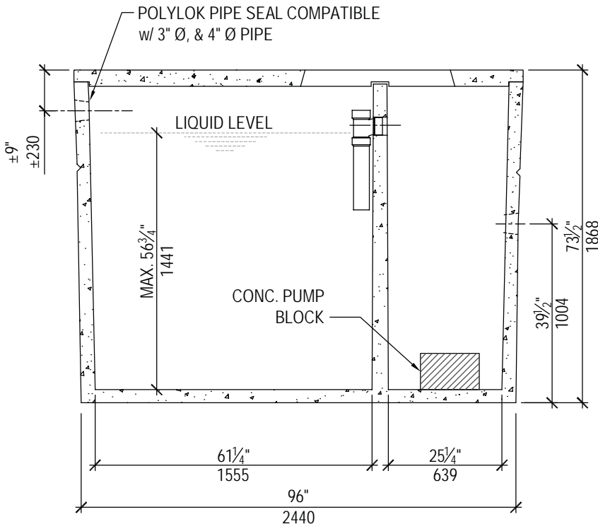
SECTION 'A'
