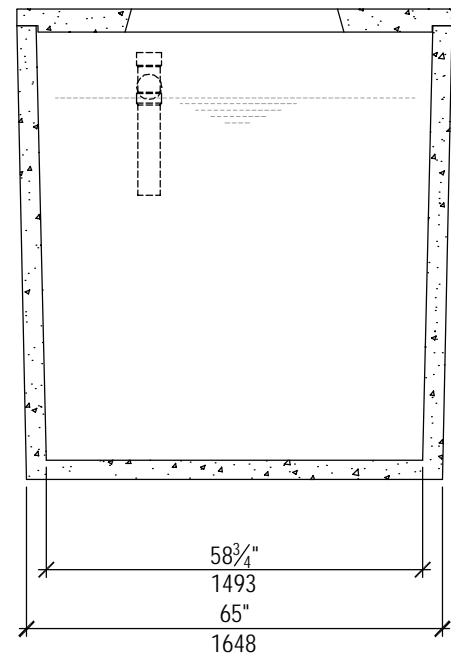
SECTION 'B'
